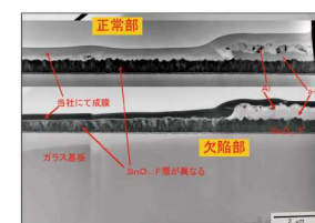
▲故障解析による断面解析画像
